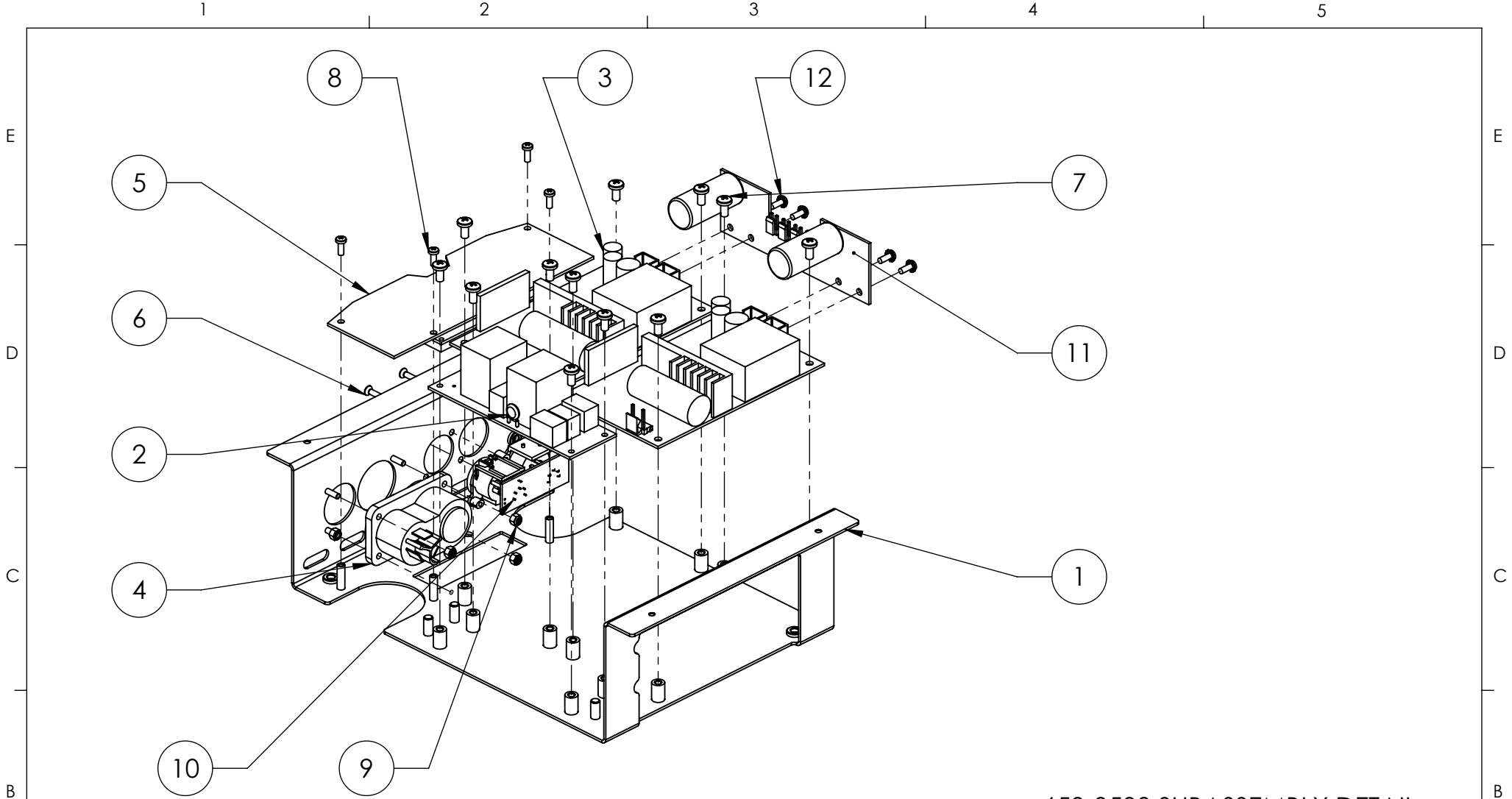
650-0500 SUBASSEMBLY DETAIL
